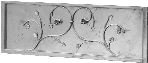
ART. 16-171-1 MISURE mm MEASURES B. 1360 - H. 425 SPESSORE mm THICK 1,5
