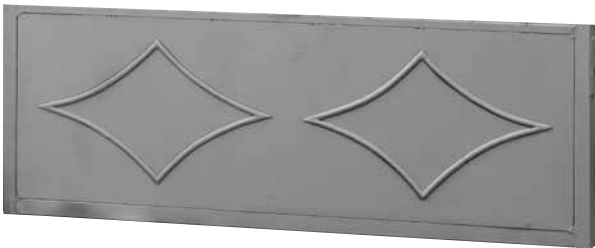
ART. 16-172-1 MISURE mm MEASURES B. 1360 - H. 425 SPESSORE mm THICK 1,5
